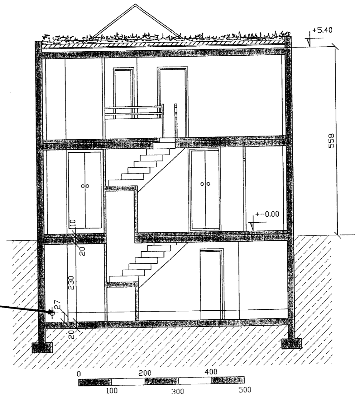
COUPE VERTICALE
