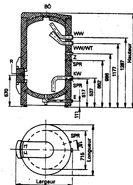
VertiCell-L de 500 litres de capacité
