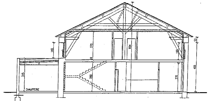
Coupe verticale ANNEXE
