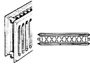
Radiateur acier 2 panneaux Epaisseur 101 mm
