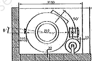
Encombrement du ballon équipé d'une station solaire DKP 6-8 et d'un vase d'expansion de 18 litres
