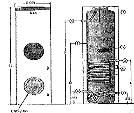
Encombrement du ballon équipé d'une station solaire DKP 6-8 et d'un vase d'expansion de 18 litres
